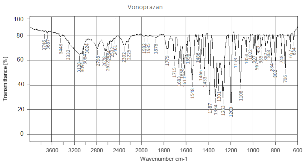
Figure 13.3: FTIR Spectra of Vonoprazan VONO
