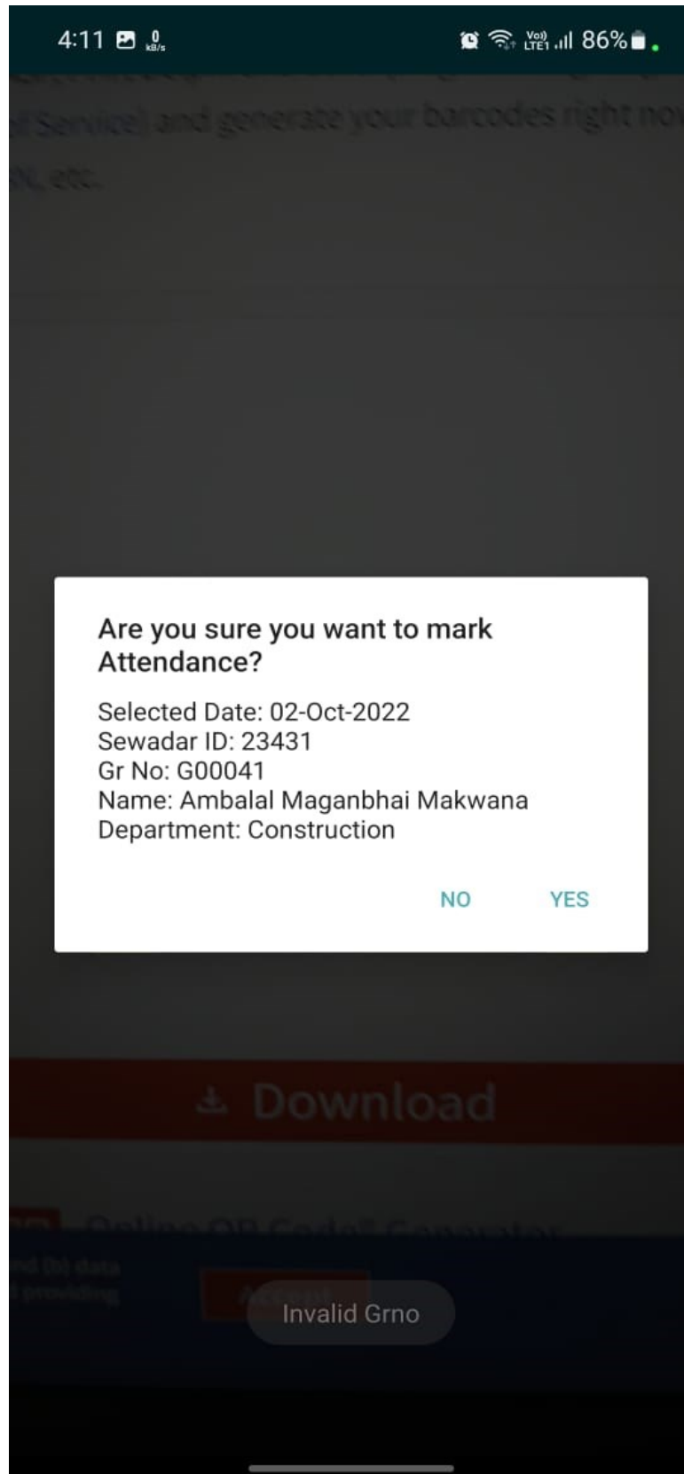
Fig.3.6.4 Fill Attendance
